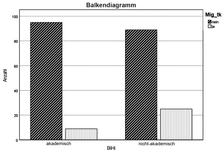
Abbildung 27. Balkendiagramm Mig_tk*BiHi.
