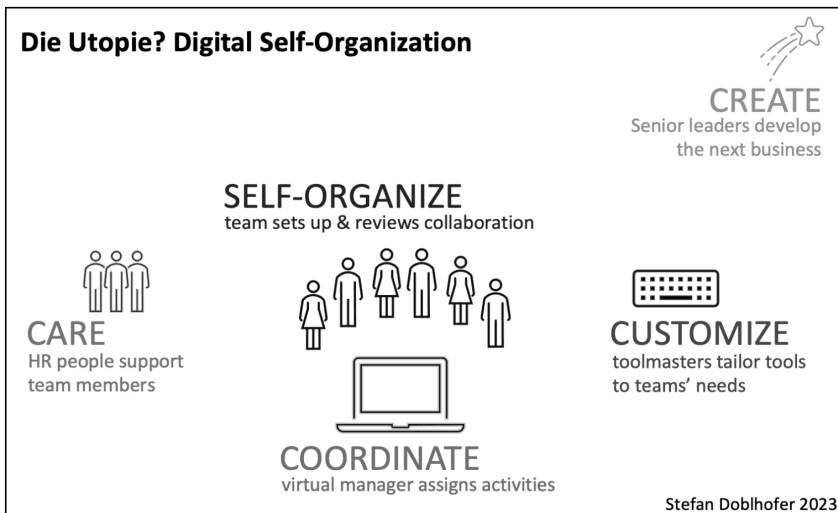
Abbildung 6: Digitale Selbstorganisation
