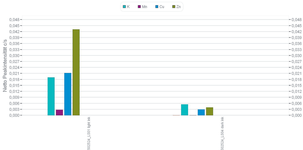
9 Diagramm: Vergleich der beiden Tinten, das Element Eisen (ausgeblendet) auf 1 normiert
