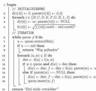
Abbildung 1: A*Algorithmus; Abbildung 2: Straßennetz im Graph modelliert (orientiert an Velden 2014)
