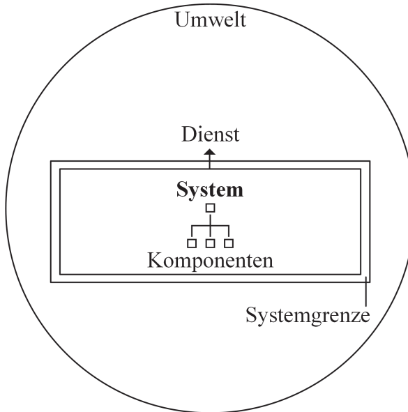
Abbildung 5: IT-System
