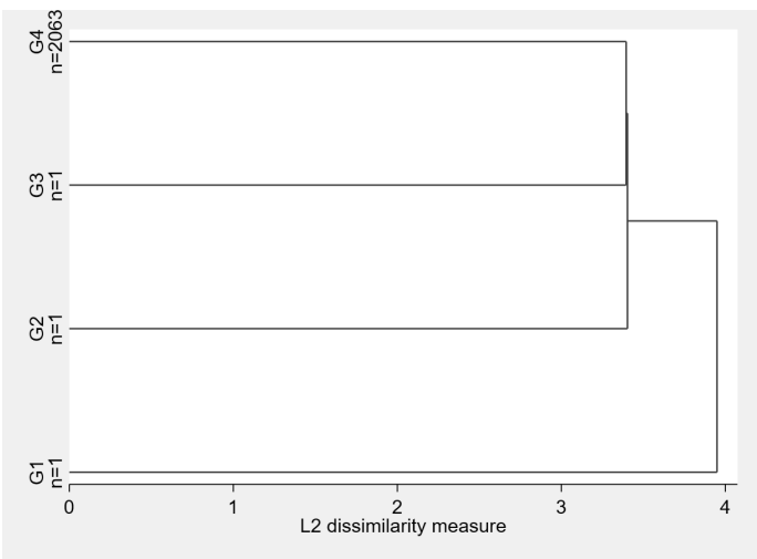
Abbildung 1: Dendrogramm Single-Linkage-Verfahren
