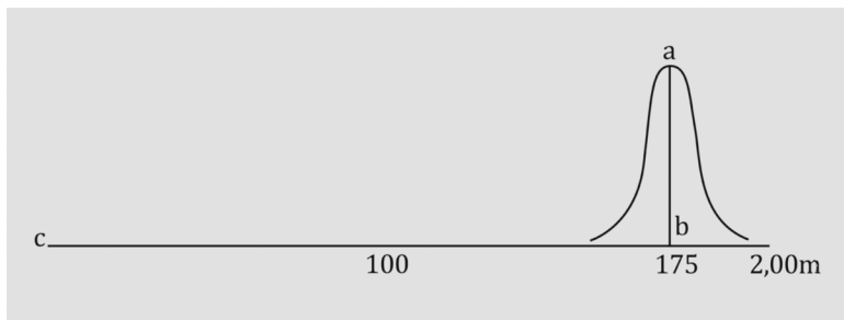
Abb. 6: Gausssche Darstellung.
