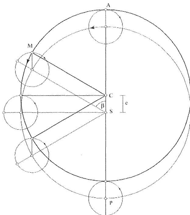
Abb. 16: Exzentrische Kreisbahn der Planeten und ihre Modellierung durch ein Epizykelmodell. Auf diese Weise wird eine einfache Kreisbahn des Mars um die Sonne durch ein epizyklisches, äquivalentes Planetenmodell dargestellt, bei dem zwei Kreise eine Überlagerung von Bewegungen als Wirkung von zwei Kräften darstellen.
