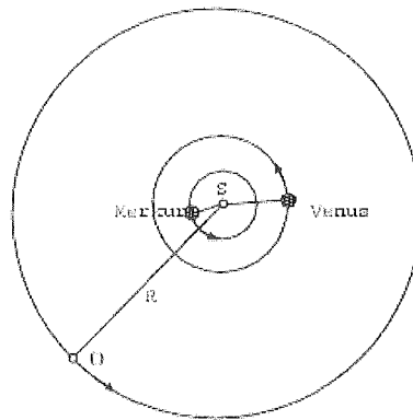
Abb. 15: Innere Planeten, heliozentrisch dargestellt.
