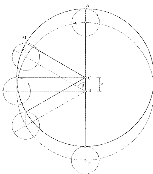
Abb. 10: Epizykalisches Modell und die Beschreibung der Bahnform mittels der Keplerschen Gesetze.
